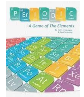
Periodic
