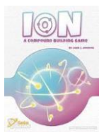
Ion
